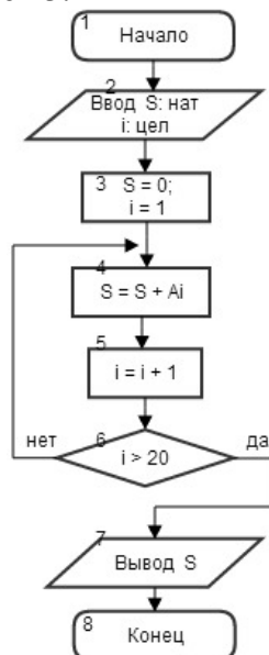
Рисунок 3 – Блок схема решения задачи 2
